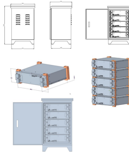
蓄電池システム IP65 防水防災仕様
